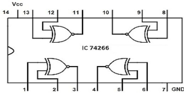
XNOR-Gate رقمه 74266.
