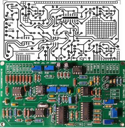
دائرة كهربية (Circuit)
